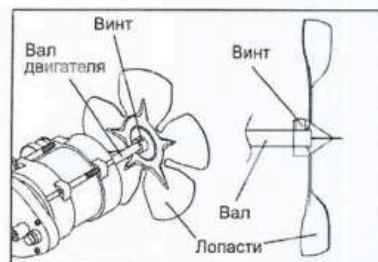
Рис 15. Снятие крыльчатки вентилятора
