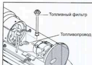
Рис. 19. Извлечение топливного фильтра
