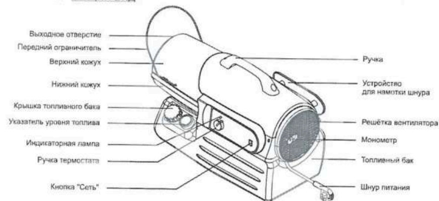
Рис. 1. KFA-70T DGP
