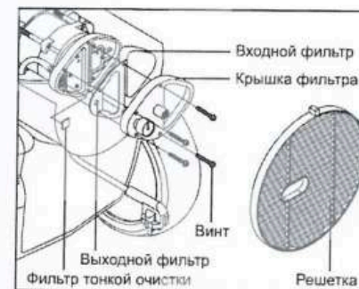
Рис. 14. Входной, выходной фильтры и фильтр тонкой очистки
