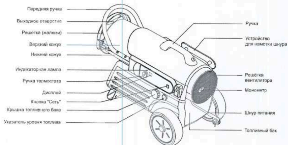
Рис. 2. KFA-125T DGP
