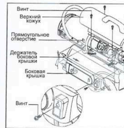
Рис. 13. Снятие верхнего кожуха
