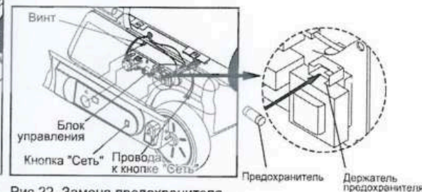
Рис 22. Замена предохранителя
