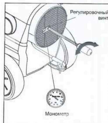
Рис. 20. Регулировка давления насоса
