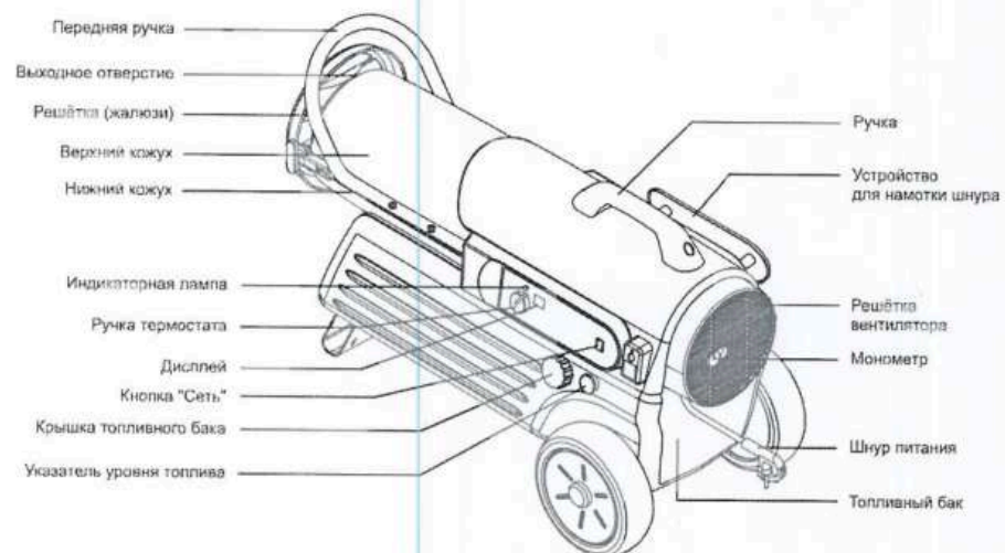
Рис. 3. KFA-170T DGP
